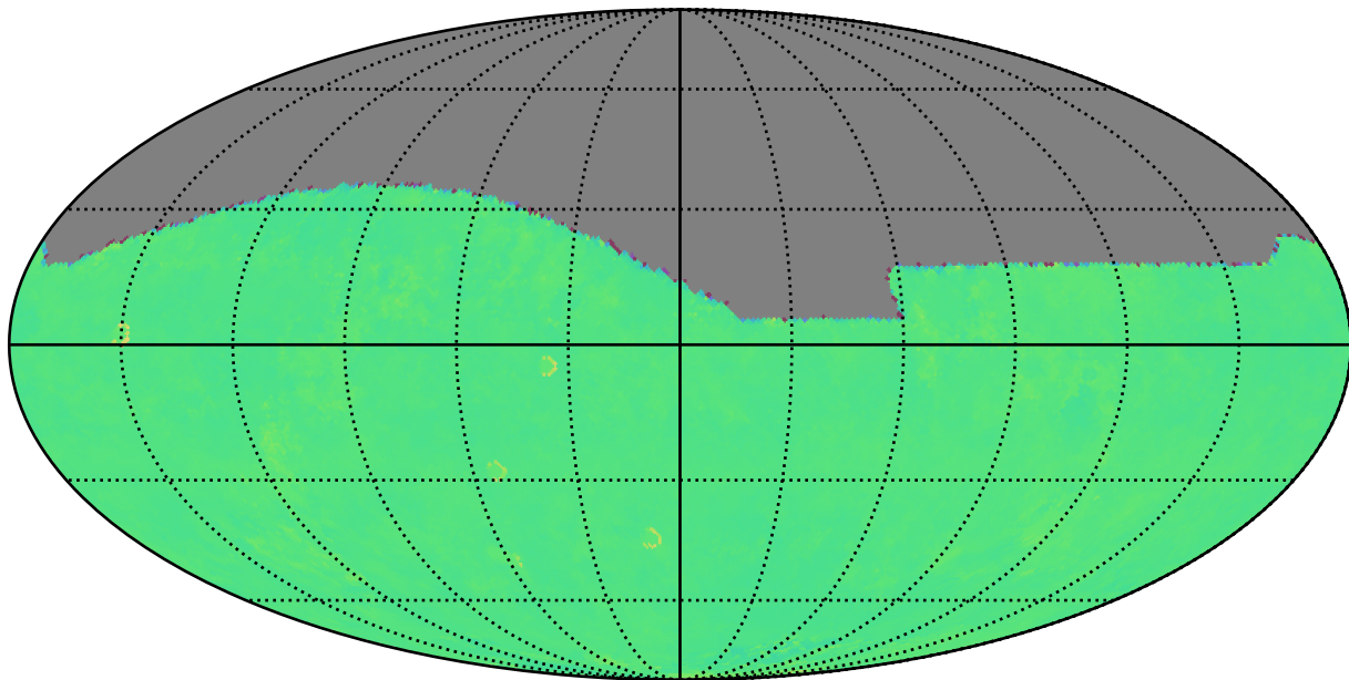
roll_pause_mjdp0_v3.4_10yrs i: Kuiper rotTelPos
