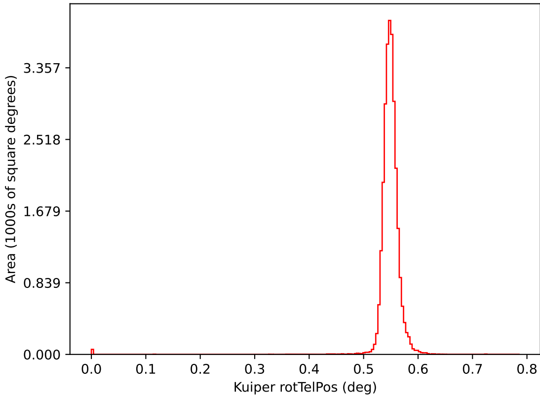
roll_pause_mjdp0_v3.4_10yrs i: Kuiper rotTelPos
