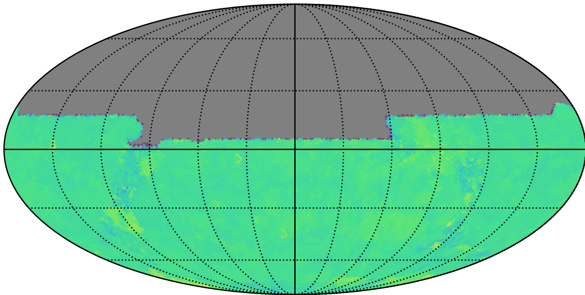
roll_mid3_const_season2v3.3_10yrs u: Kuiper rotTelPos
