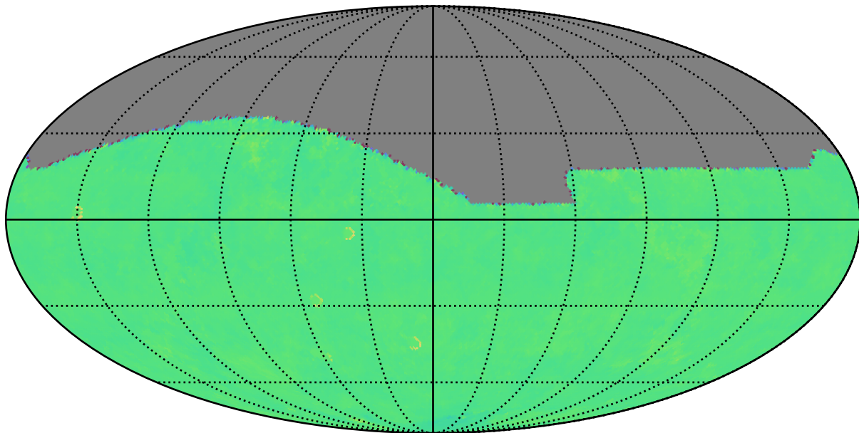
roll_mid3_const_season2v3.3_10yrs i: Kuiper rotTelPos
