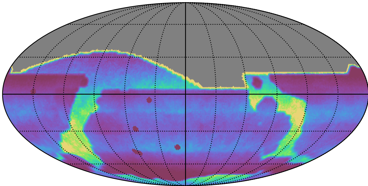
roll_mid3_const_season2v3.3_10yrs : DCRprecision
