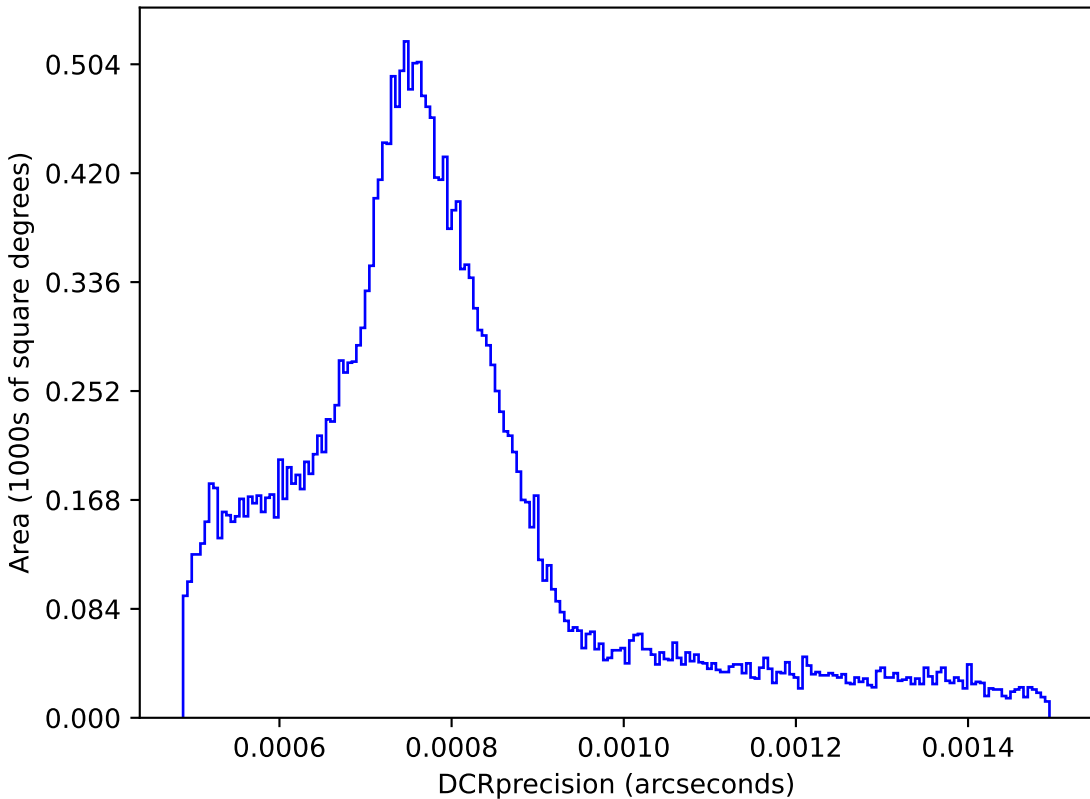
roll_mid3_const_season2v3.3_10yrs : DCRprecision
