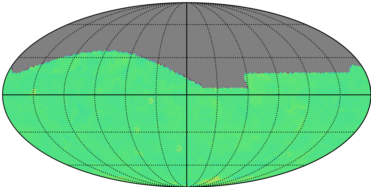
roll_mid2_const_season_v3.3_10yrs r: Kuiper rotTelPos
