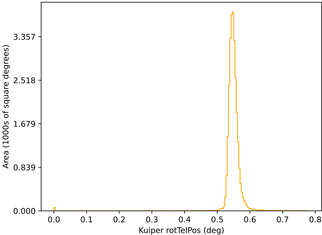
roll_mid2_const_season_v3.3_10yrs r: Kuiper rotTelPos
