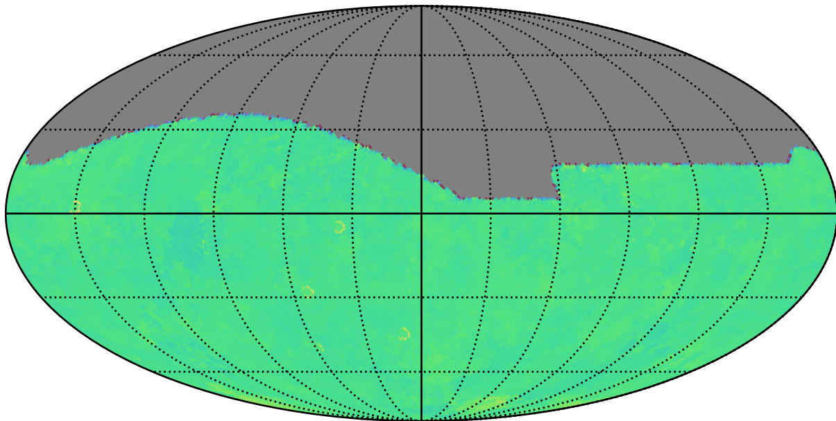
roll_mid2_const_season_v3.3_10yrs g: Kuiper rotTelPos
