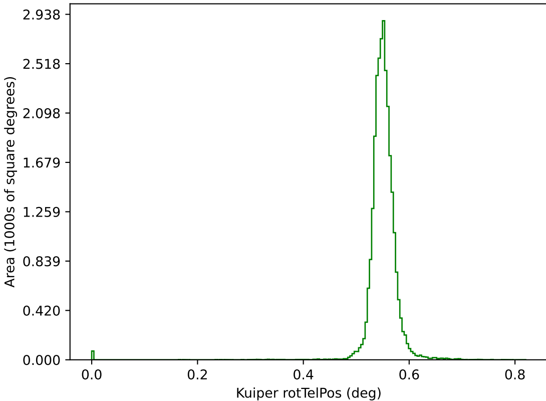
roll_mid2_const_season_v3.3_10yrs g: Kuiper rotTelPos
