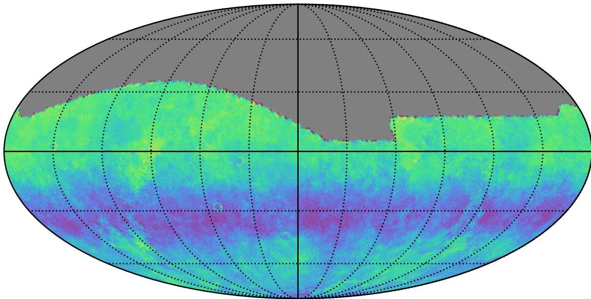
roll_mid2_const_season_v3.3_10yrs g: Kuiper rotSkyPos
