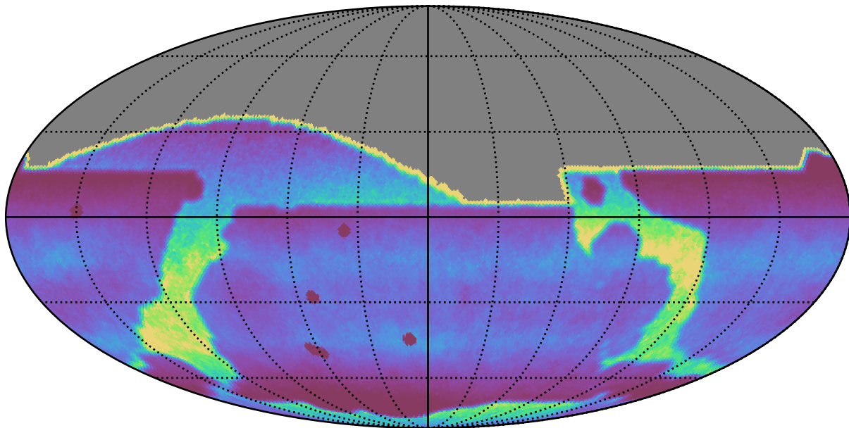
roll_mid2_const_season_v3.3_10yrs : DCRprecision
