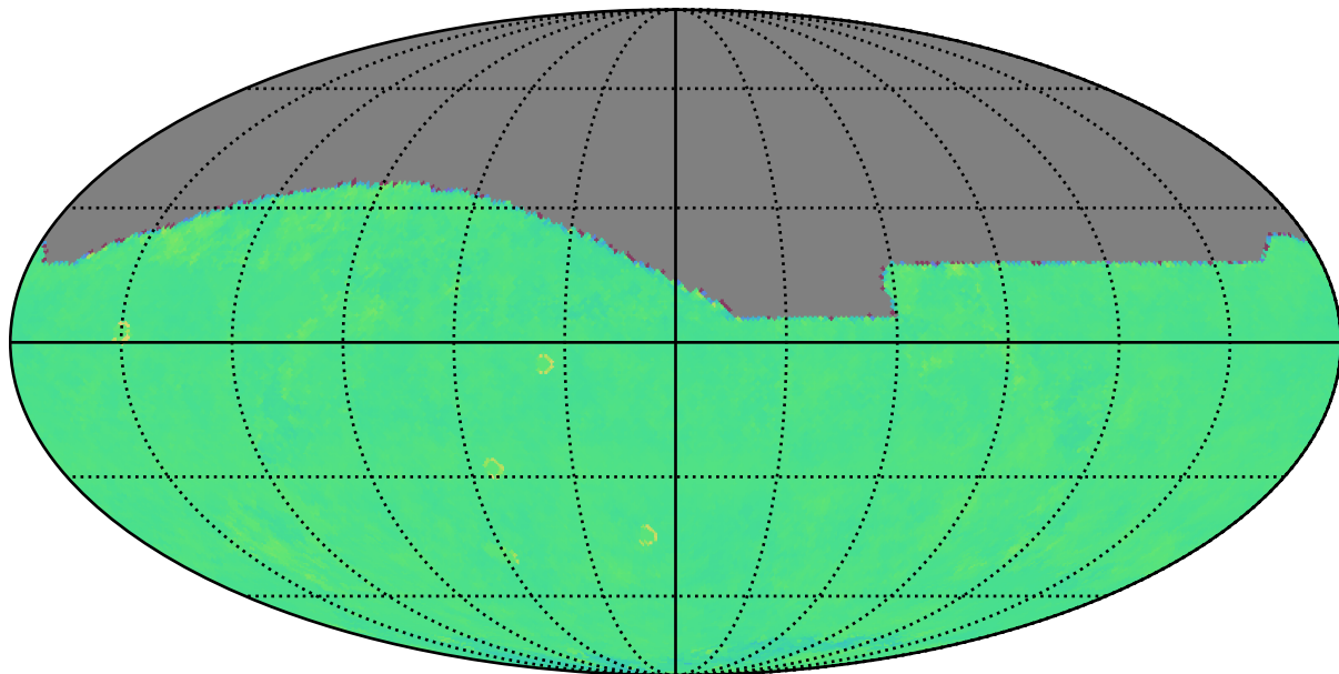
roll_mid2_const_season6v3.3_10yrs z: Kuiper rotTelPos
