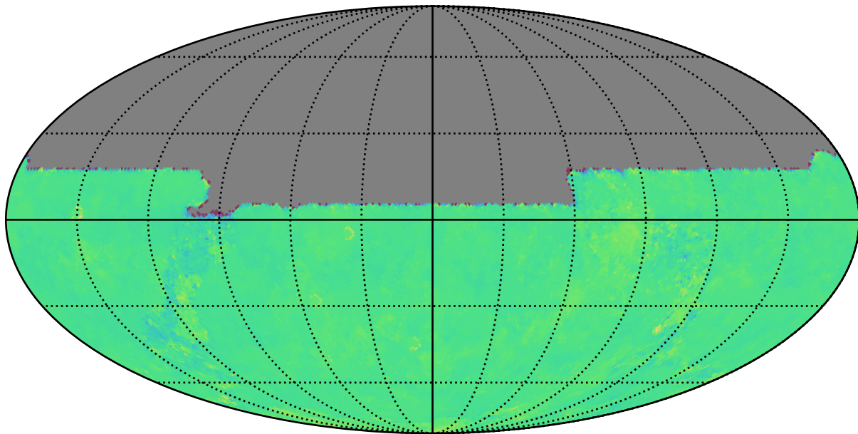
roll_mid2_const_season6v3.3_10yrs u: Kuiper rotTelPos
