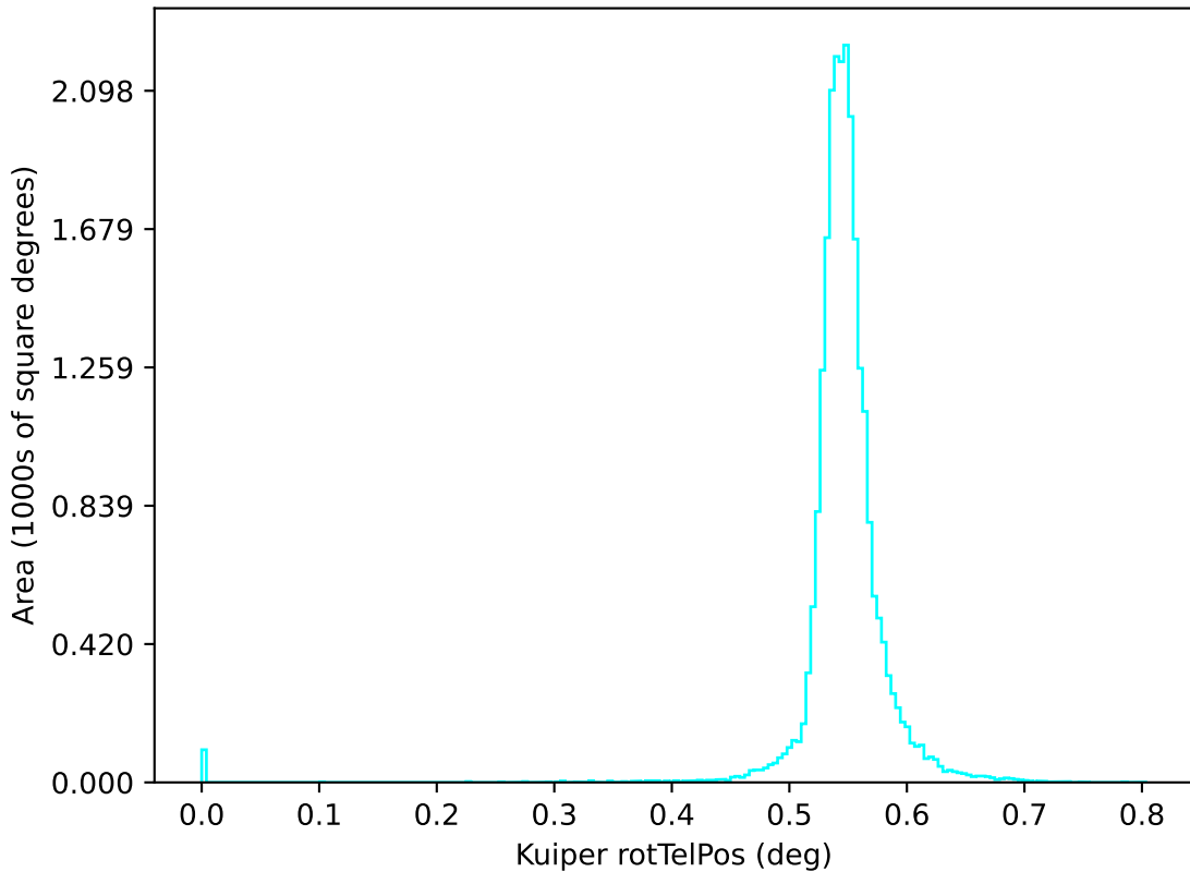
roll_mid2_const_season6v3.3_10yrs u: Kuiper rotTelPos
