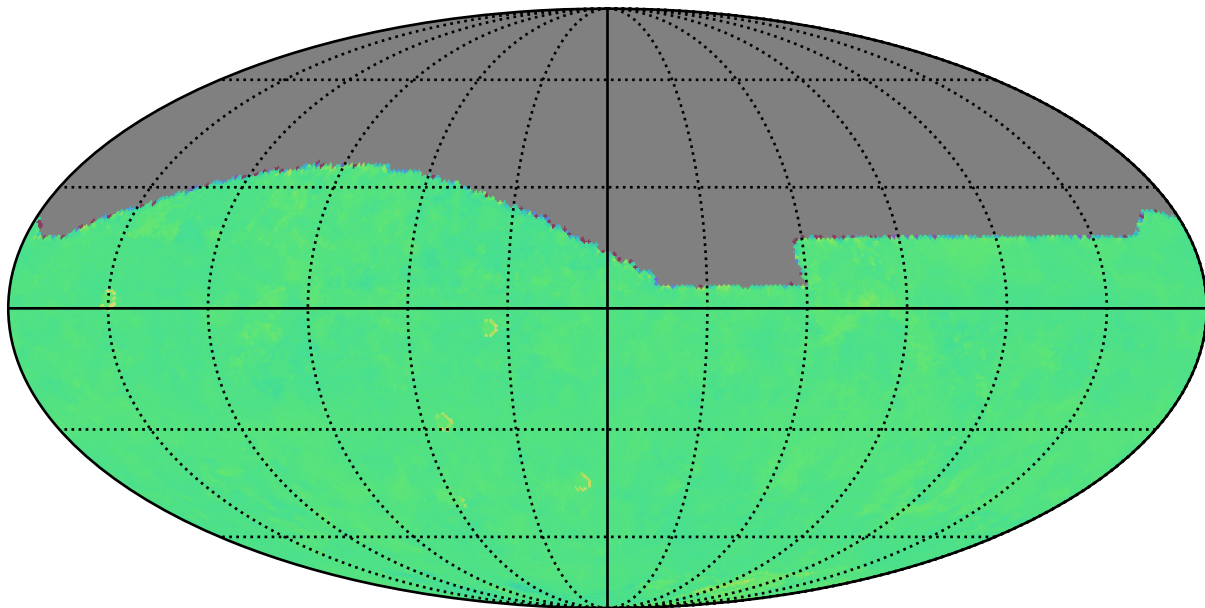
roll_mid2_const_season6v3.3_10yrs i: Kuiper rotTelPos
