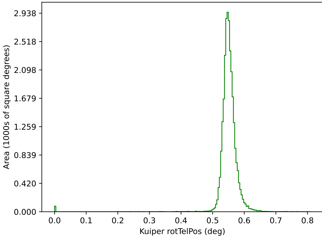
roll_mid2_const_season6v3.3_10yrs g: Kuiper rotTelPos
