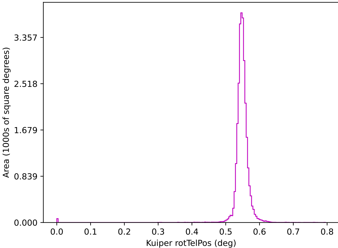
roll_mid1_const_season4v3.3_10yrs z: Kuiper rotTelPos
