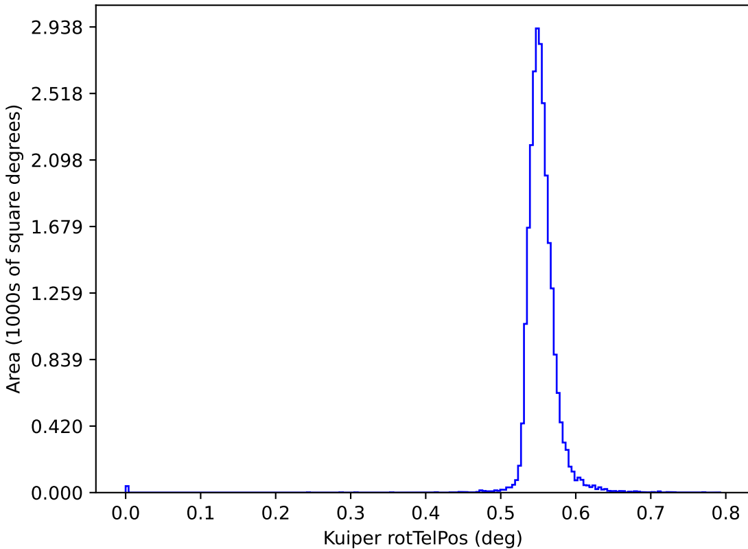
roll_mid1_const_season4v3.3_10yrs y: Kuiper rotTelPos
