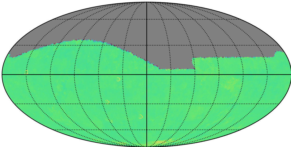
roll_mid1_const_season4v3.3_10yrs r: Kuiper rotTelPos
