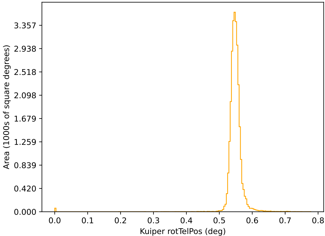
roll_mid1_const_season4v3.3_10yrs r: Kuiper rotTelPos
