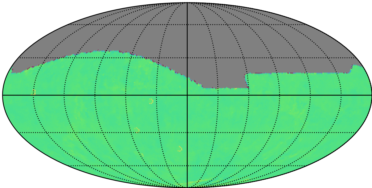
roll_mid1_const_season4v3.3_10yrs i: Kuiper rotTelPos
