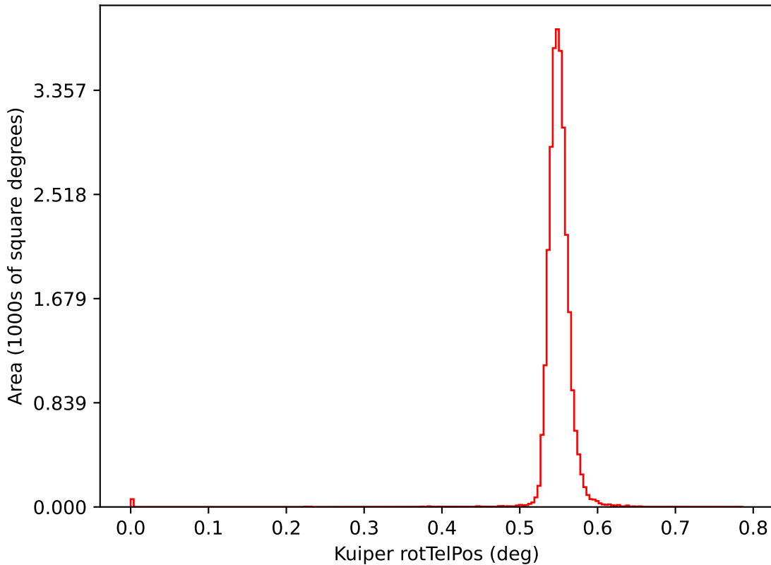
roll_mid1_const_season4v3.3_10yrs i: Kuiper rotTelPos
