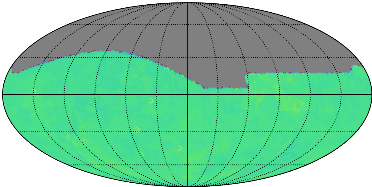
roll_mid1_const_season4v3.3_10yrs g: Kuiper rotTelPos
