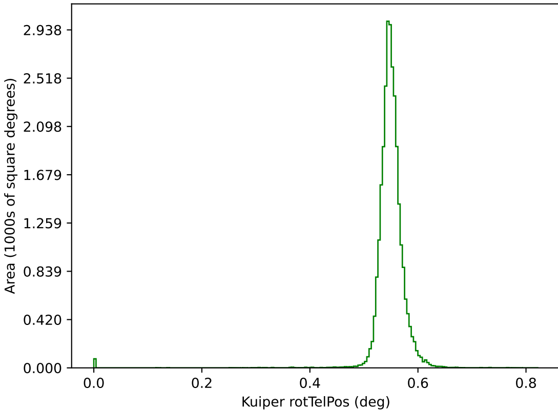
roll_mid1_const_season4v3.3_10yrs g: Kuiper rotTelPos
