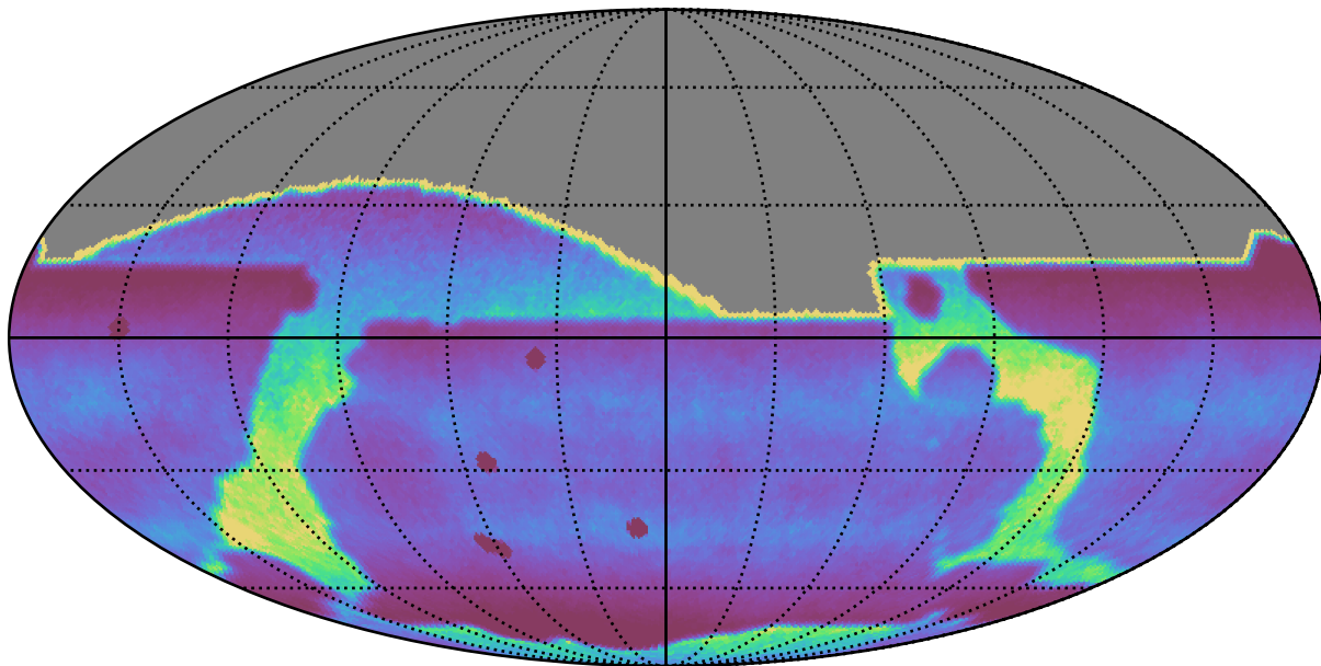
roll_mid1_const_season4v3.3_10yrs : DCRprecision
