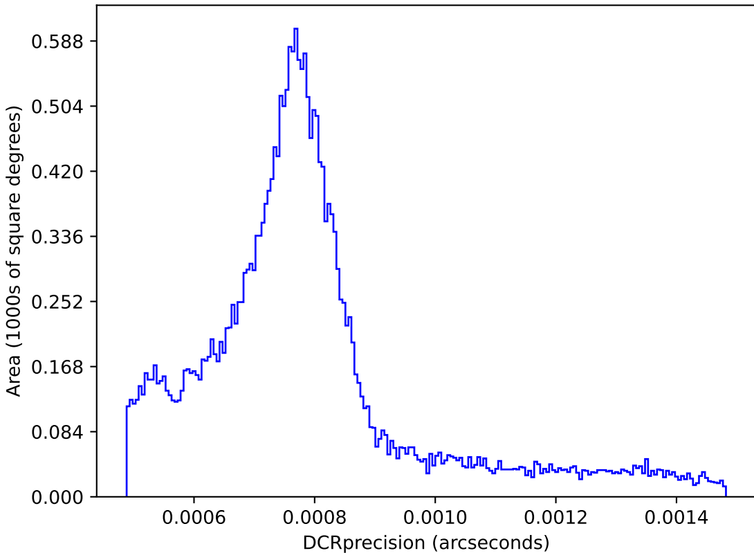
roll_mid1_const_season4v3.3_10yrs : DCRprecision
