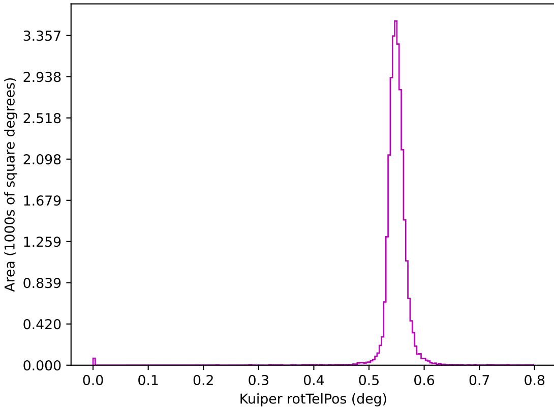
roll_mid1_const_season2v3.3_10yrs z: Kuiper rotTelPos
