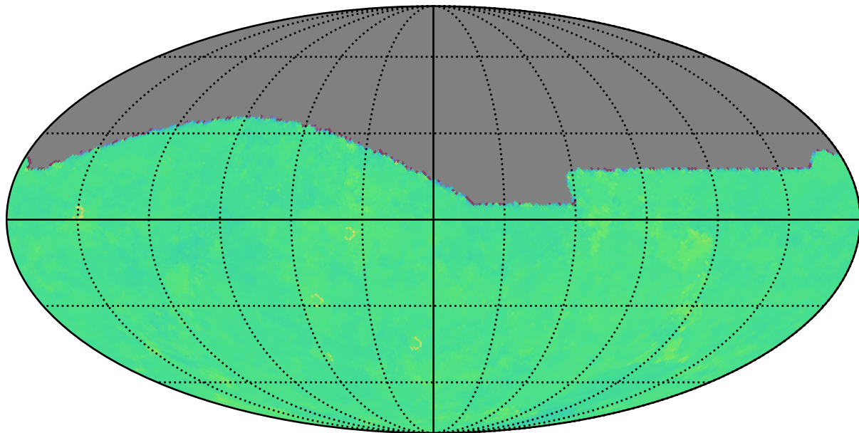
roll_mid1_const_season2v3.3_10yrs g: Kuiper rotTelPos
