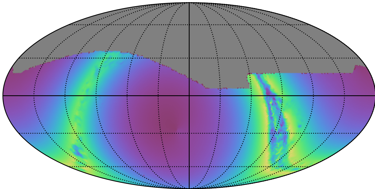
roll_3_v3.4_10yrs : young_stars
