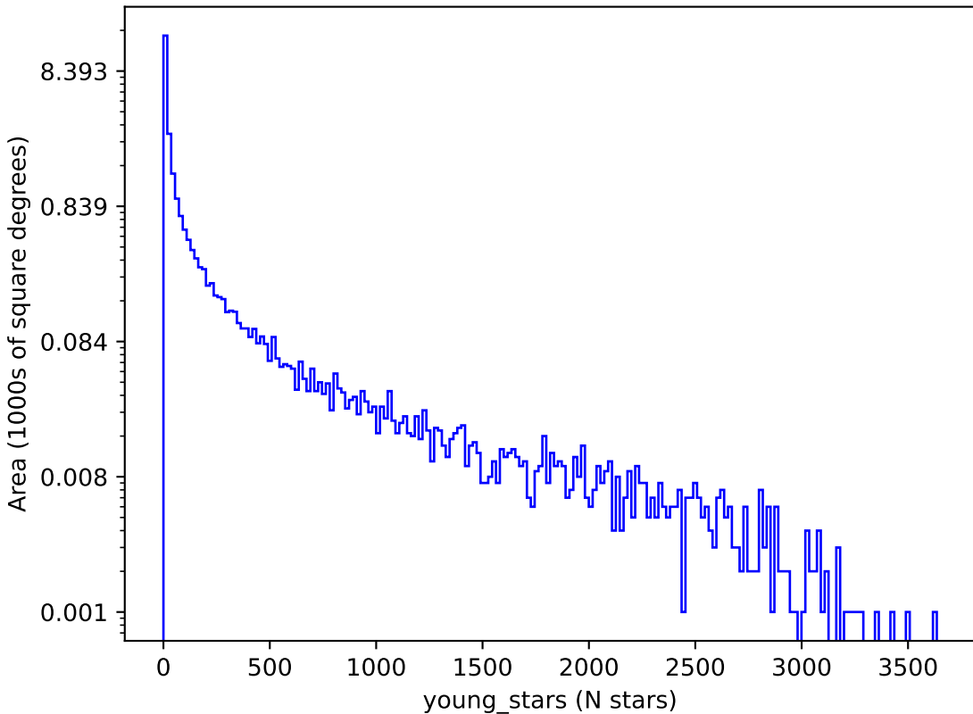
roll_3_v3.4_10yrs : young_stars
