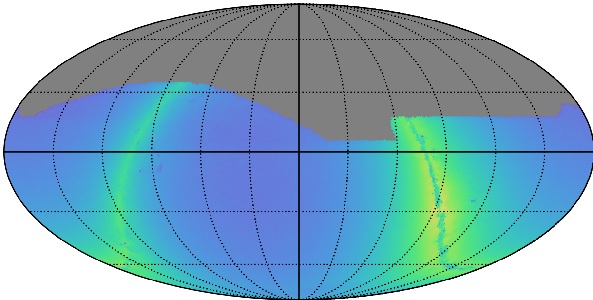
roll_3_v3.4_10yrs z: Nstars_no_crowding
