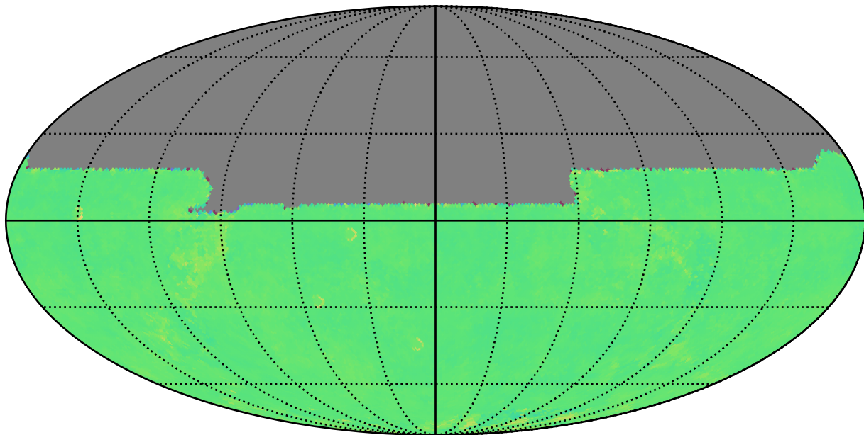
roll_3_v3.4_10yrs y: Kuiper rotTelPos
