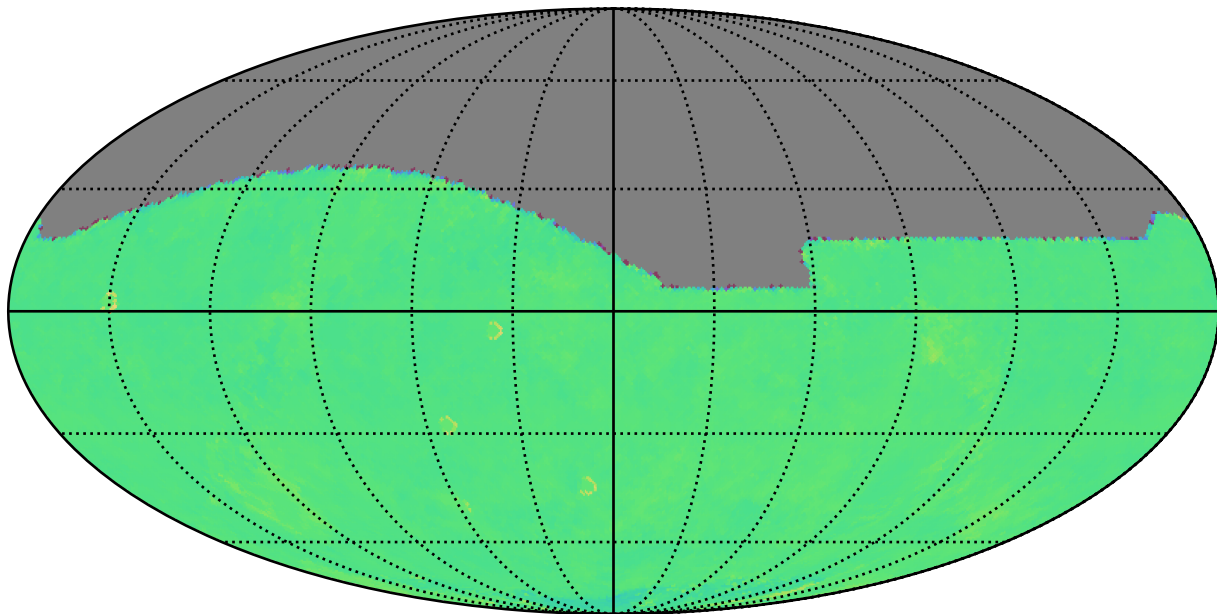
roll_3_v3.4_10yrs r: Kuiper rotTelPos
