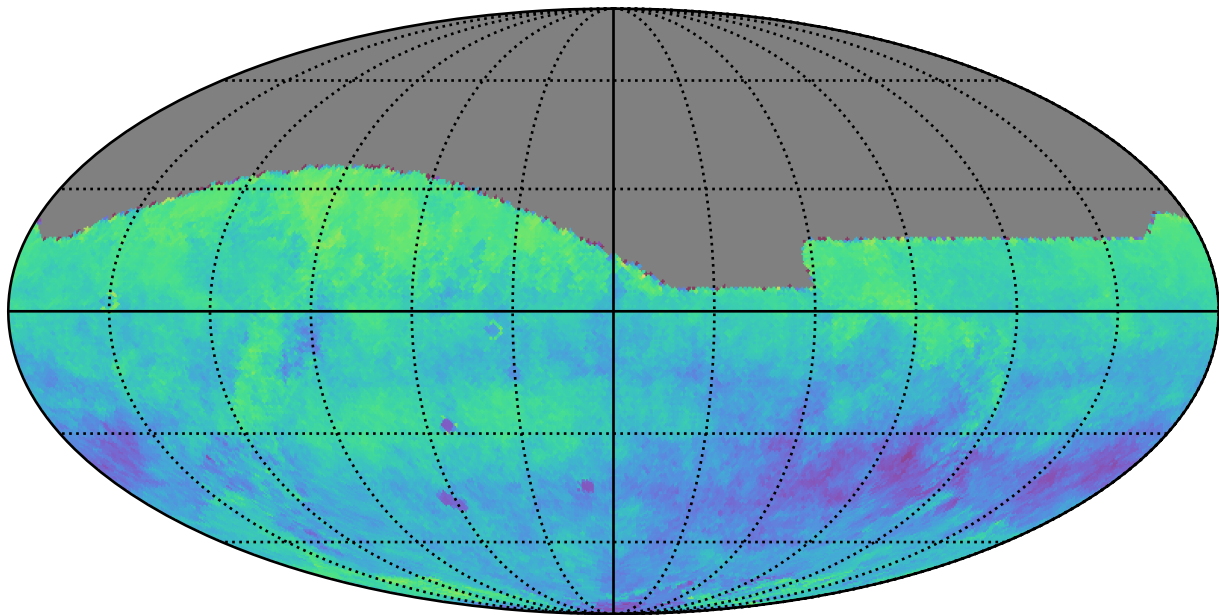
roll_3_v3.4_10yrs z: Kuiper rotSkyPos
