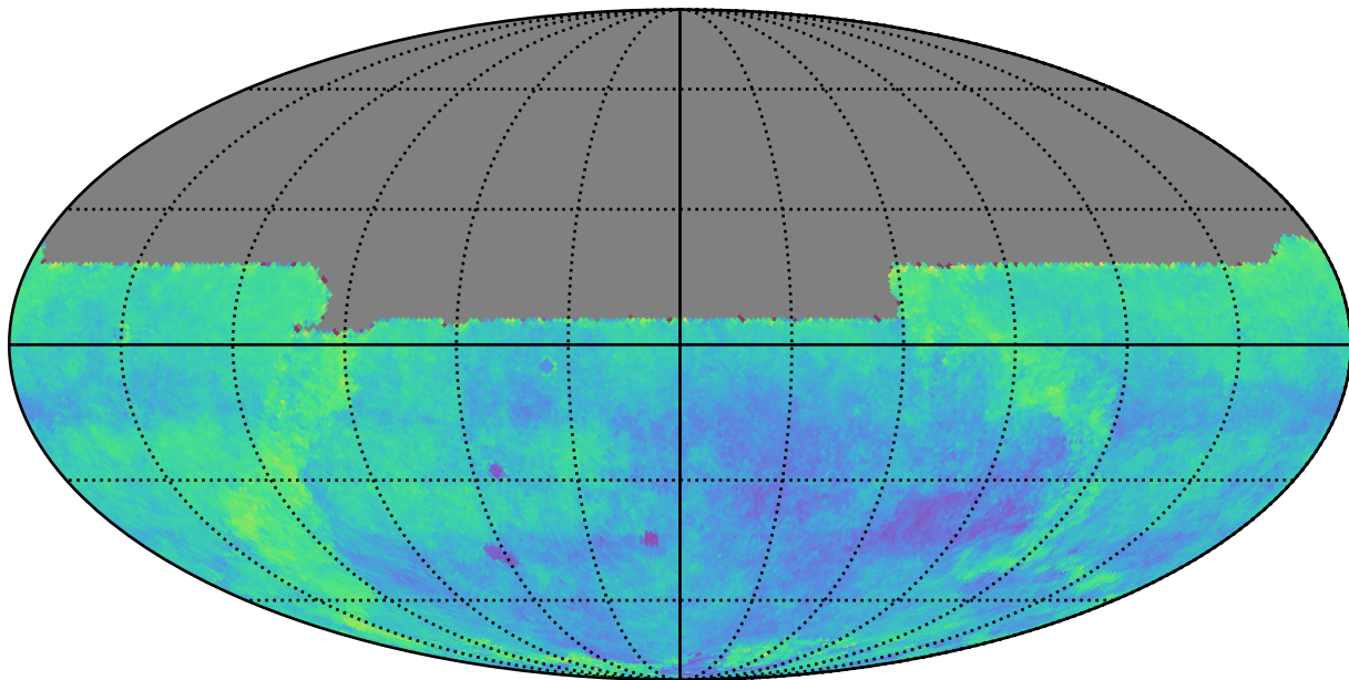
roll_3_v3.4_10yrs y: Kuiper rotSkyPos
