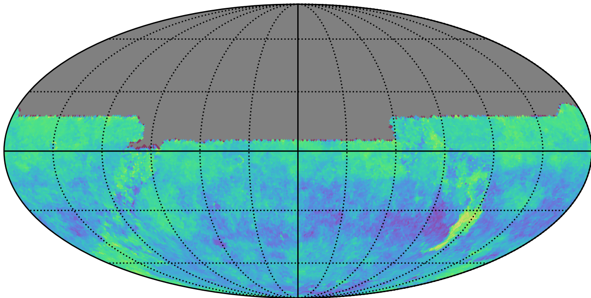
roll_3_v3.4_10yrs u: Kuiper rotSkyPos
