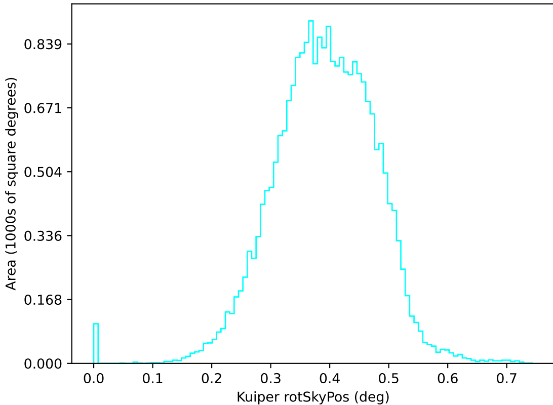
roll_3_v3.4_10yrs u: Kuiper rotSkyPos
