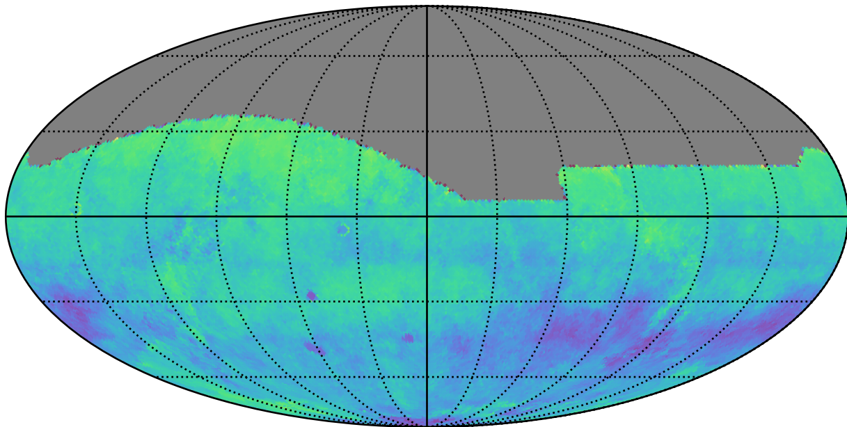
roll_3_v3.4_10yrs i: Kuiper rotSkyPos
