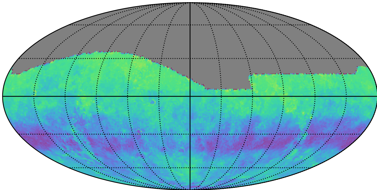
roll_3_v3.4_10yrs g: Kuiper rotSkyPos
