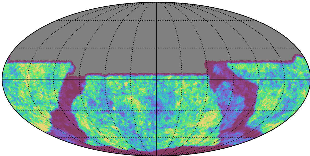
roll_3_v3.4_10yrs y band: Gaps_24hr
