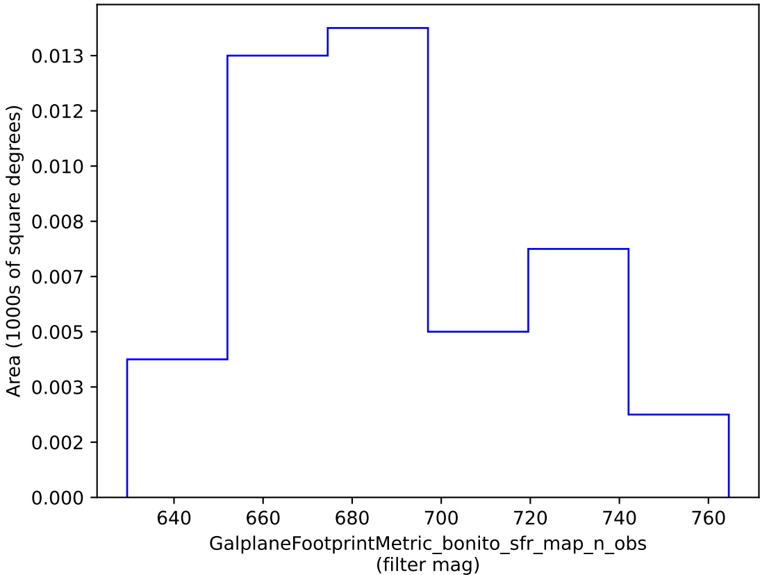
roll_3_v3.4_10yrs : GalplaneFootprintMetric_bonito_sfr_map_n_obs
