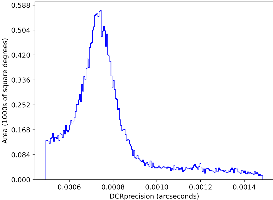
roll_3_v3.4_10yrs : DCRprecision
