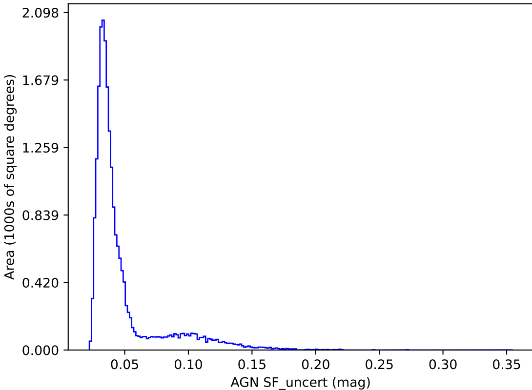
roll_3_v3.4_10yrs y band: AGN SF_uncert
