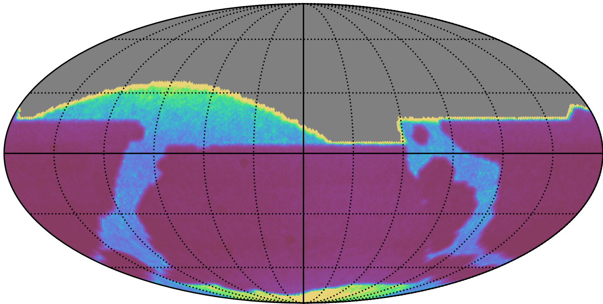
roll_3_v3.4_10yrs : properMotion
