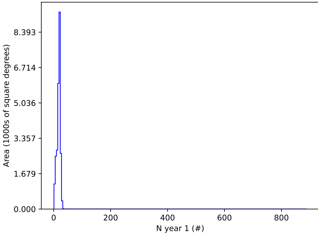
roll_3_v3.4_10yrs y and night < 365: N year 1
