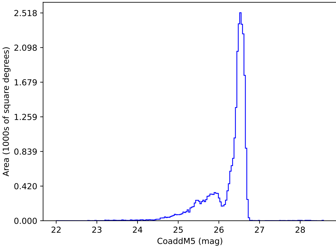
roll_3_v3.4_10yrs i: CoaddM5
