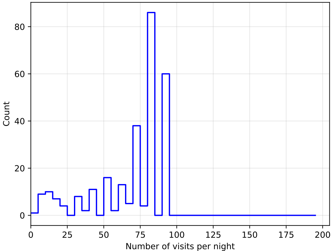
roll_3_v3.4_10yrs all bands: DD:ELAISS1 NVisitsPerNight
