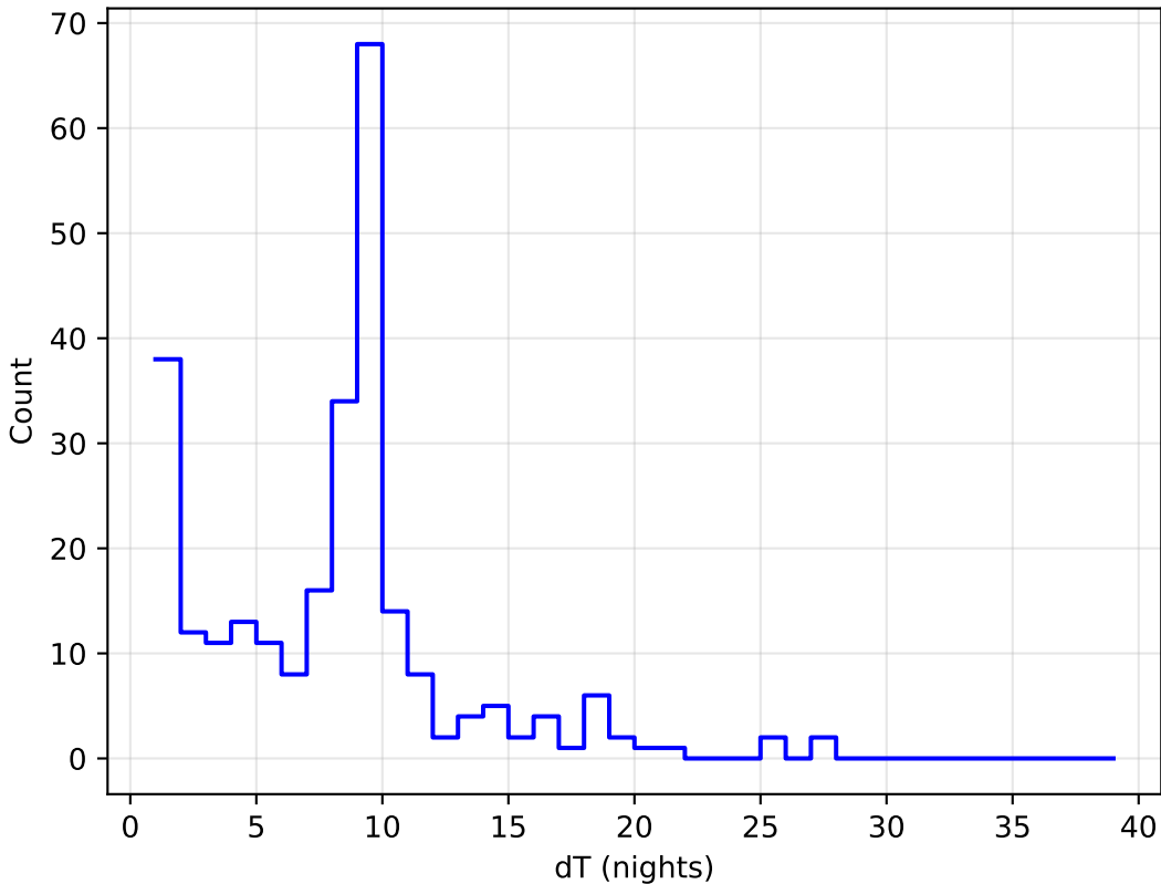
roll_3_v3.4_10yrs all bands: DD:ELAISS1 Delta Nights Histogram
