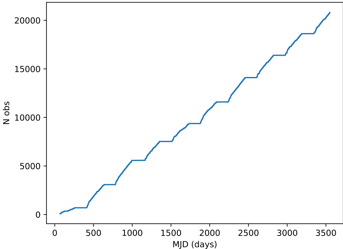
roll_3_v3.4_10yrs all bands: DD:ELAISS1 Cumulative NVisits
